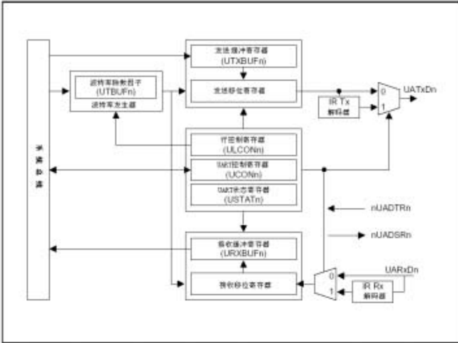
图 6.2.2 串行口功能模块。
