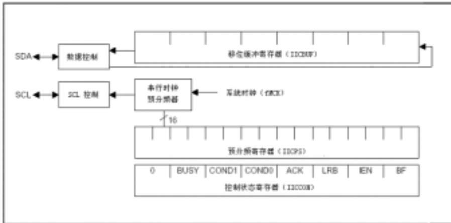
图 6.2.6 S3C4510B IIC 总线控制器的功能模块图
