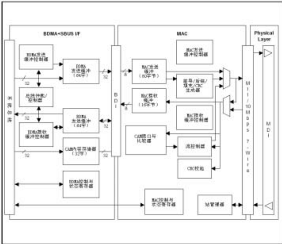
图 6.2.9 为以太网系统的流控框图。
