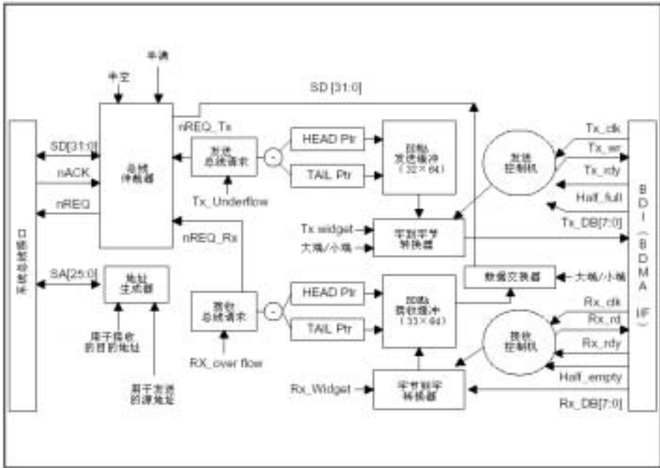
图 6.2.13 BDMA 控制模块图
