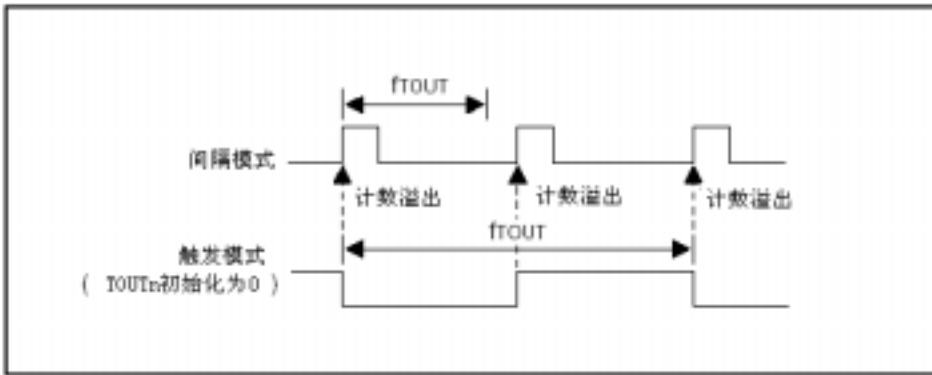
图 6.2.3 定时器输出信号时序
