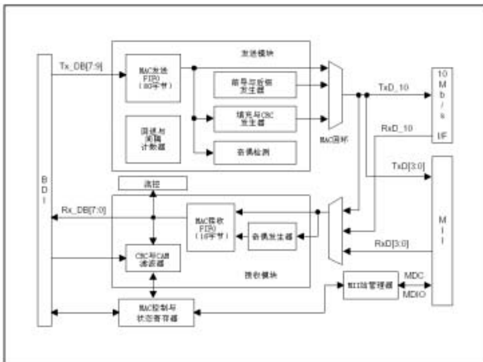
图 6.2.10 MAC 层流控功能模块
