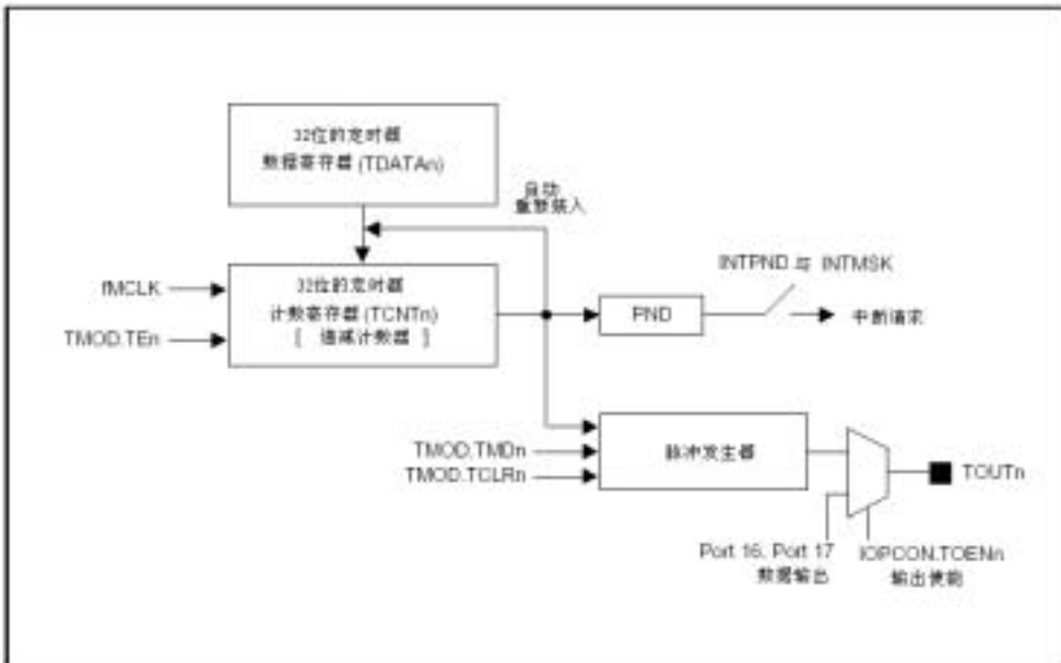
图 6.2.4 定时器的功能模块图
