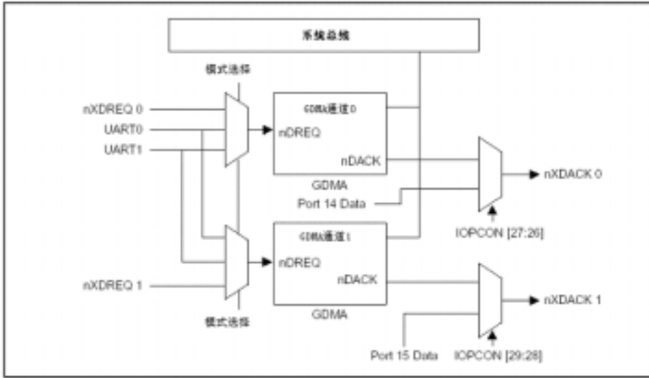
图 6.2.5 GDMA 控制器的功能模块图
