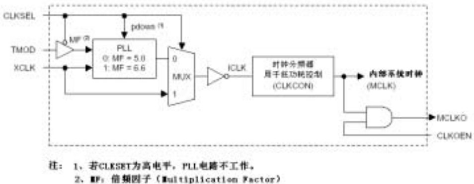
图 5.2.7 系统时钟电路
